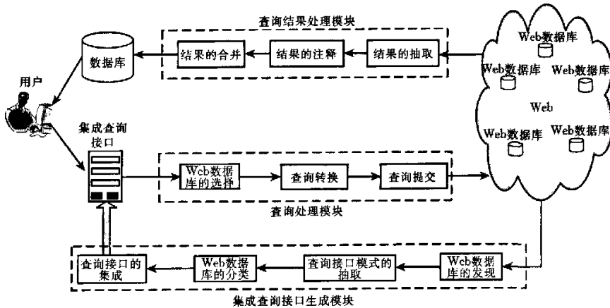
图 3 Deep Web 数据集成框架
